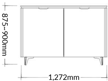
2 Door (587mm)
