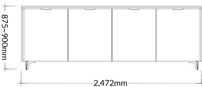
4 Door (587mm)
