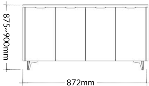
4 Door (387mm)
