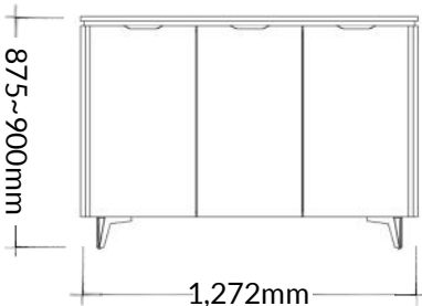
3 Door (387mm)
